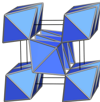
Stishovit (Rutil-Tyo)
