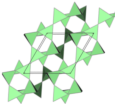
Coesit
