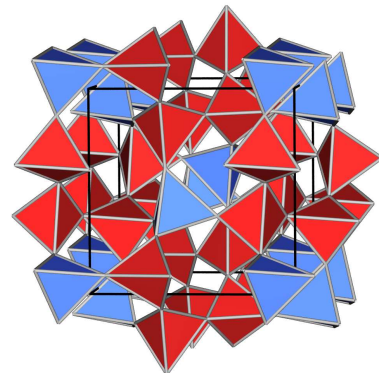
Keatit
