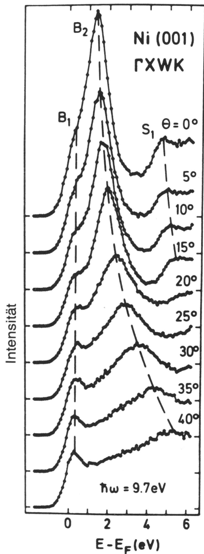
Winkelaufgelöste Ni-IPE-Spektren
