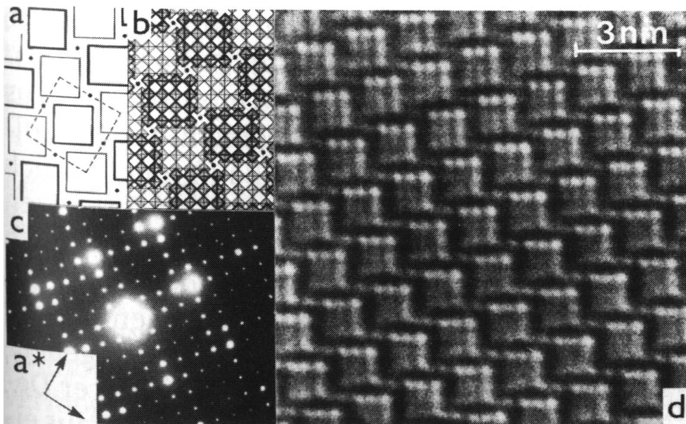
TEM-Bilder der Blockstruktur von Nb_{4/4}[Nb_{13}W_3O_{44}]
