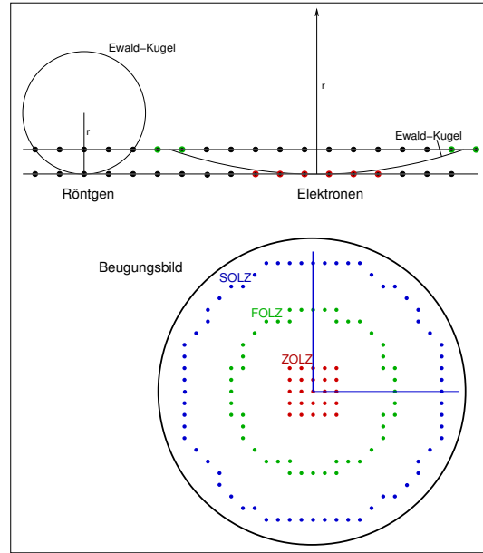
Ewald-Konstruktion: Vergleich zwischen Röntgen- und e^- -Beugung
