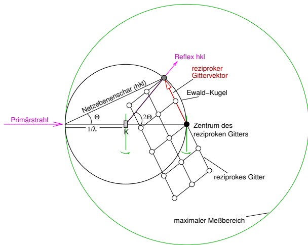
Ewald-Konstruktion zur Beschreibung der Beugung
