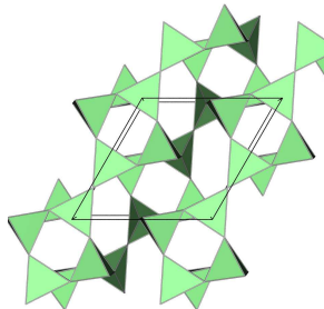
Coesit
