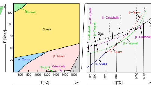
p-T-Diagramm
