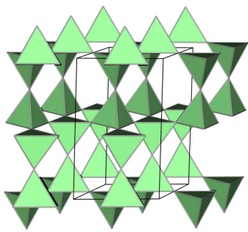
Tridymit
