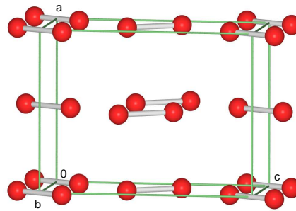
Kristallstruktur von I 2
