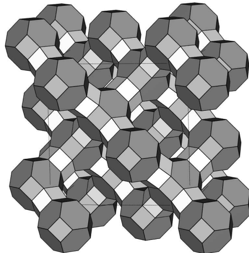
Faujasit
