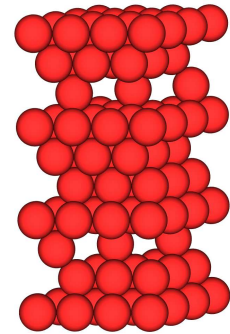
β-Alumina
