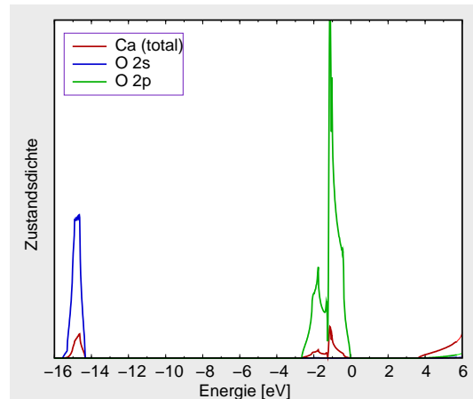
CaO (Ionenkristall)
