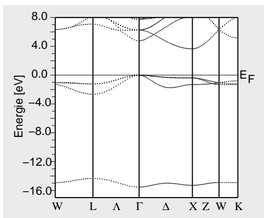
CaO (Ionenkristall)
